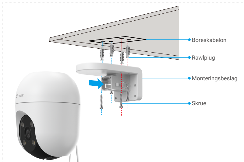
Fig. 1 Montering i loft
