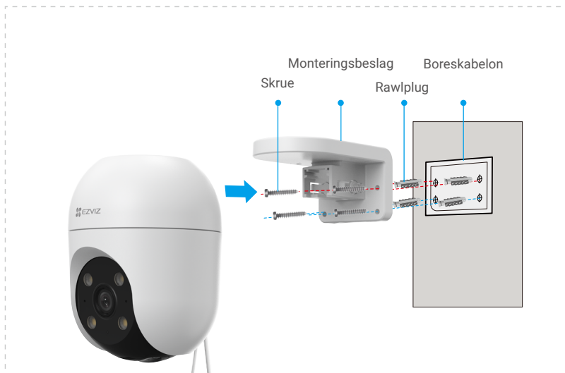
Fig. 2 Montering på væg
